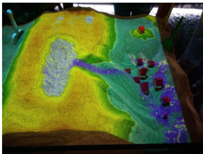
FIGURA 1: Uso da SARndbox pra simulação de rompimento de barragem. Fonte: próprio autor, 2019.
